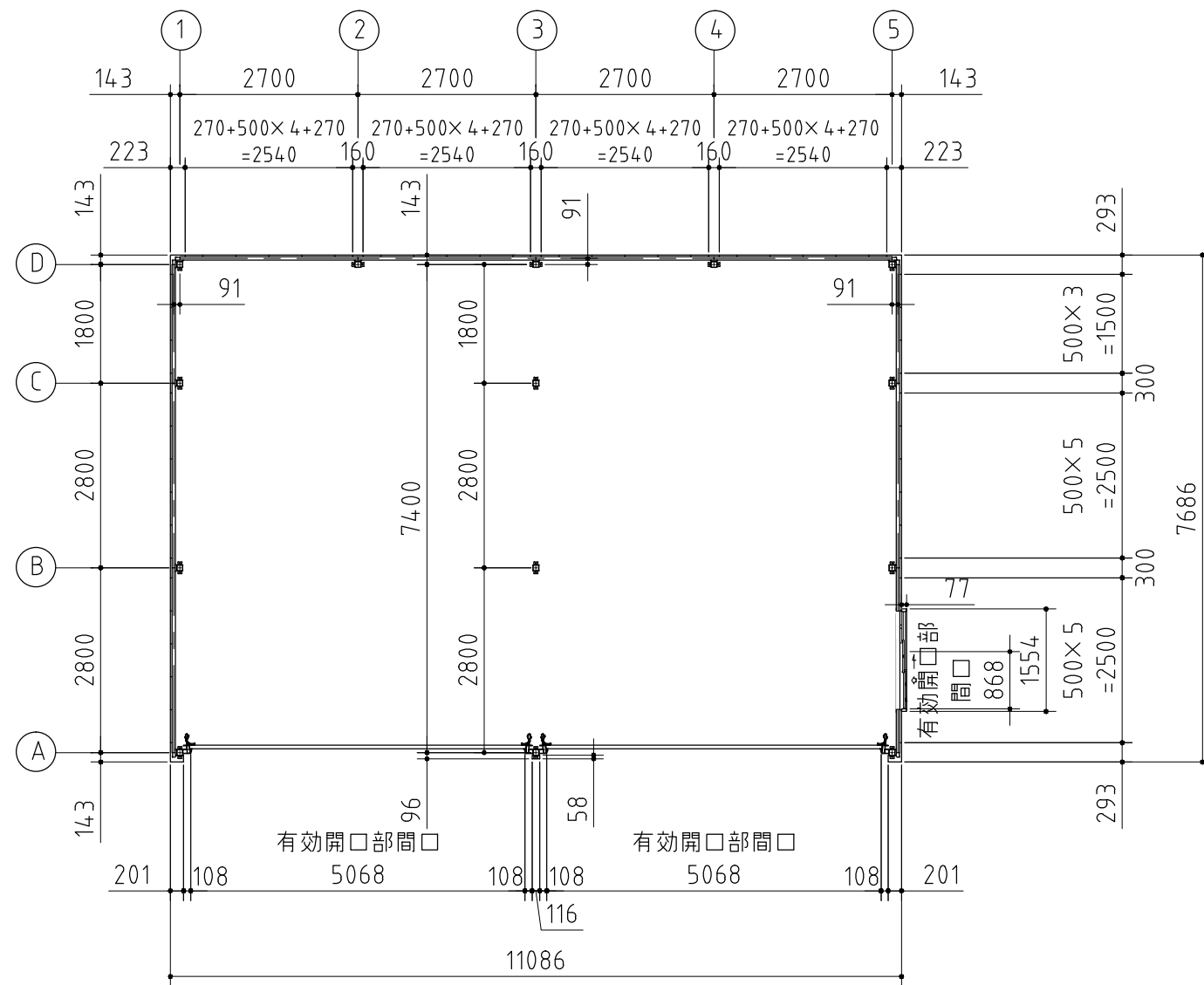
平面図
